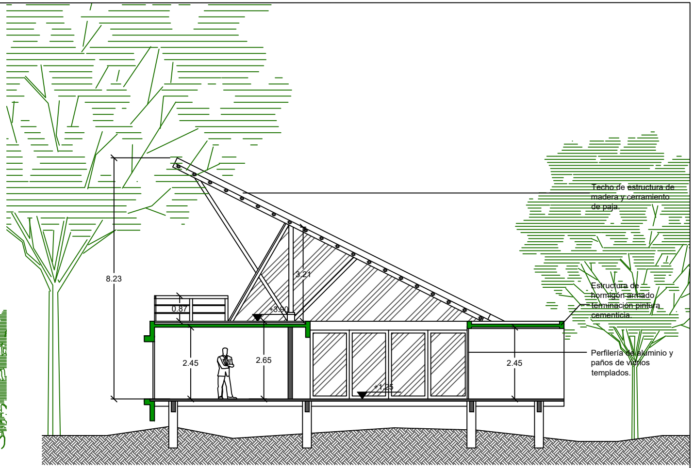
Corte Transversal
