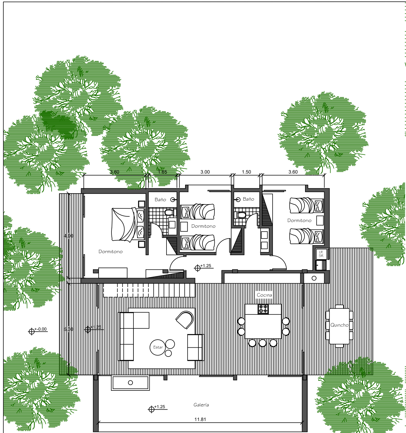
Planta Equipada Vivienda de 3 Dormitorios
